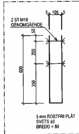
DETALJ A 1:10
